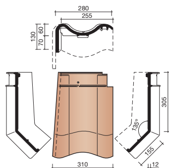
7280 LINKER GEVELKNIKPAN
