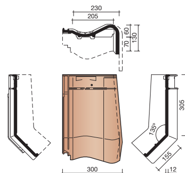
7290 RECHTER GEVELKNIKPAN
