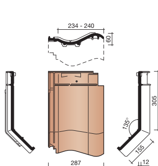
8200 KNIKPAN
