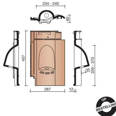
8728 DAKDOORVOER INCL. AANSL. Ø 125 MM
