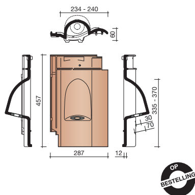
8741 DAKDOORVOER INCL. AANSL. Ø 100 MM
