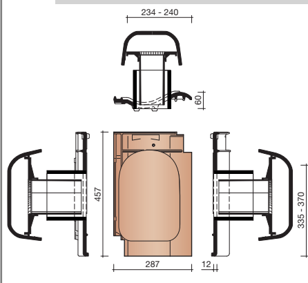
8728 DAKDOORVOER INCL. AANSL. Ø 125 MM
