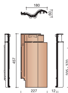
8030 DRIEKWART PAN
