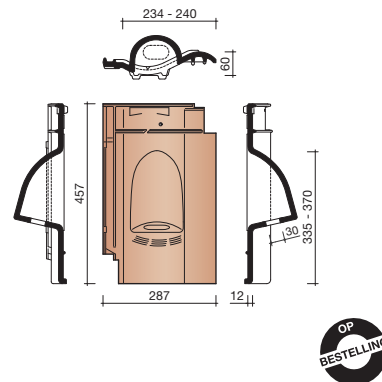
8660 GIERZWALUWPAN
