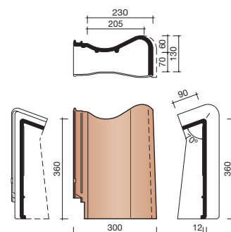
7590 RECHTER GEVELCHAPERONPAN
