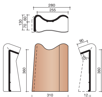
7580 LINKER GEVELCHAPERONPAN
