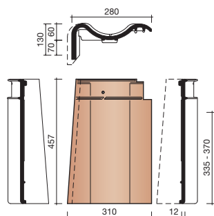
7080 LINKER GEVELPAN
