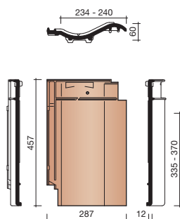
0000 MADURA DAKPAN
