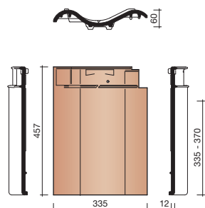
8050 PAN MET DUBBELE WEL
