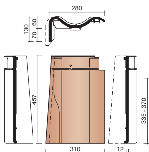
8545 GEVELAANSLUITPAN LINKS
