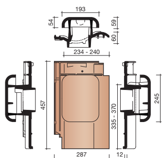
8741 DAKDOORVOER INCL. AANSL. Ø 100 MM
