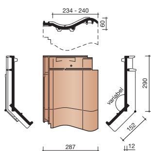
8200 KNIKPAN OP MAAT (VERLIJMD)
