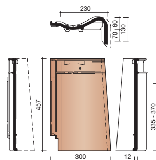
7090 RECHTER GEVELPAN
