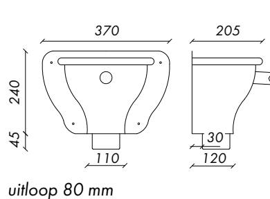
Afbeelding 1.54: Vergaarbak Haarlem
