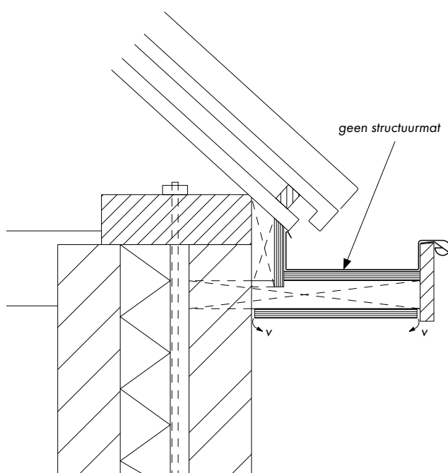
Afbeelding 1.3: buitenliggende omtimmerde goot
