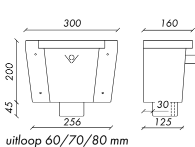
Afbeelding 1.53: Vergaarbak Vierkant
