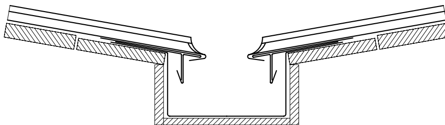
Afbeelding 1.5: verdiepte kilgoot
