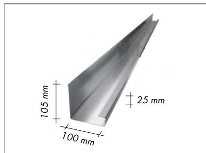
Afbeelding 1.8: verholen goot, 3 meter
