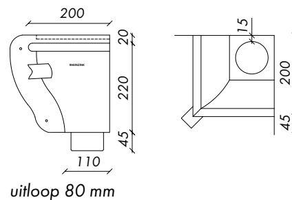
Afbeelding 1.60: Vergaarbak Haarlem hoekmodel
