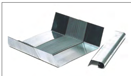
Afbeelding 1.35: RHEINZINK-expansie-element met kraalstuk
