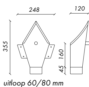
Afbeelding 1.57: Vergaarbak Trechter
