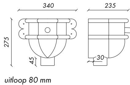
Afbeelding 1.58: Vergaarbak Louvre
