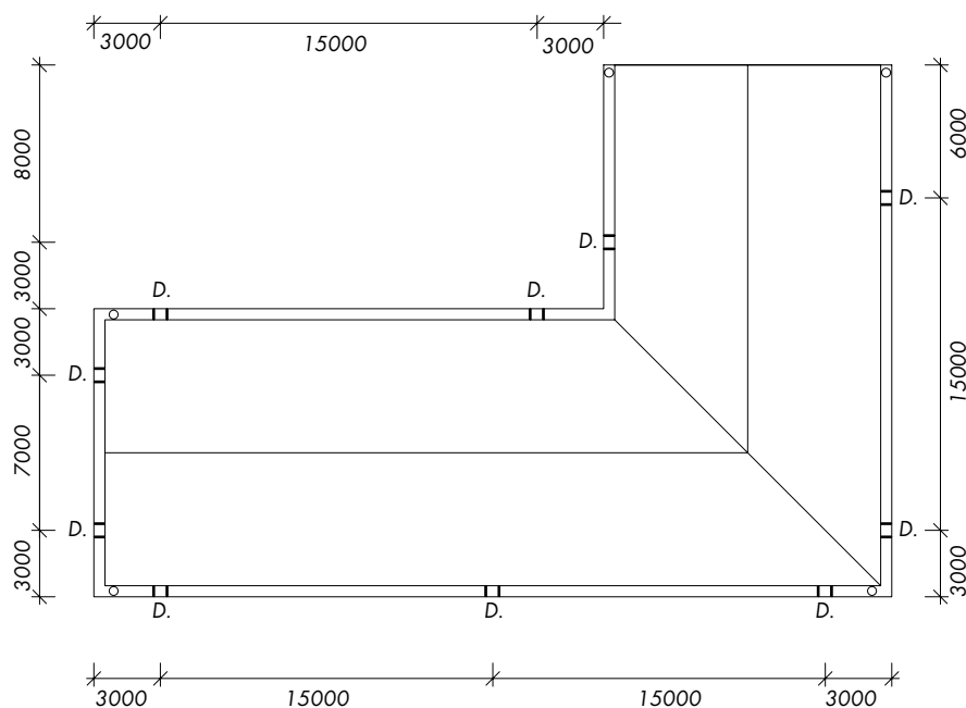
Afbeelding 1.31: bovenaanzicht positionering van de dilatatie van een vrijhangende goot (maten in mm)
