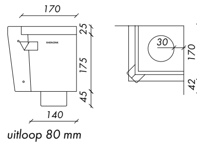
Afbeelding 1.59: Vergaarbak Vierkant hoekmodel
